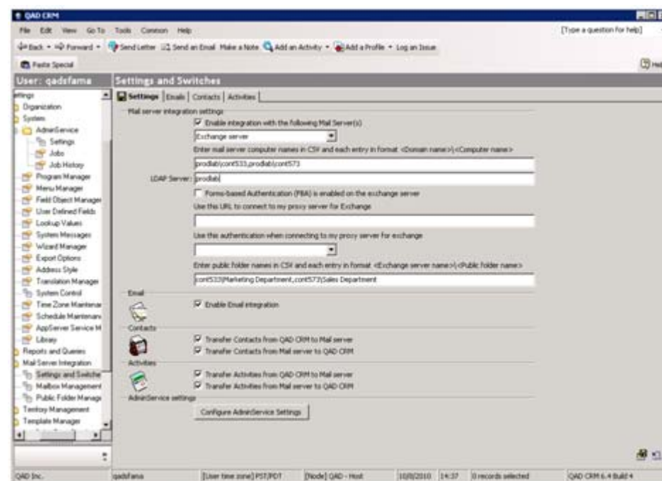
Fig. 14.24 Settings
