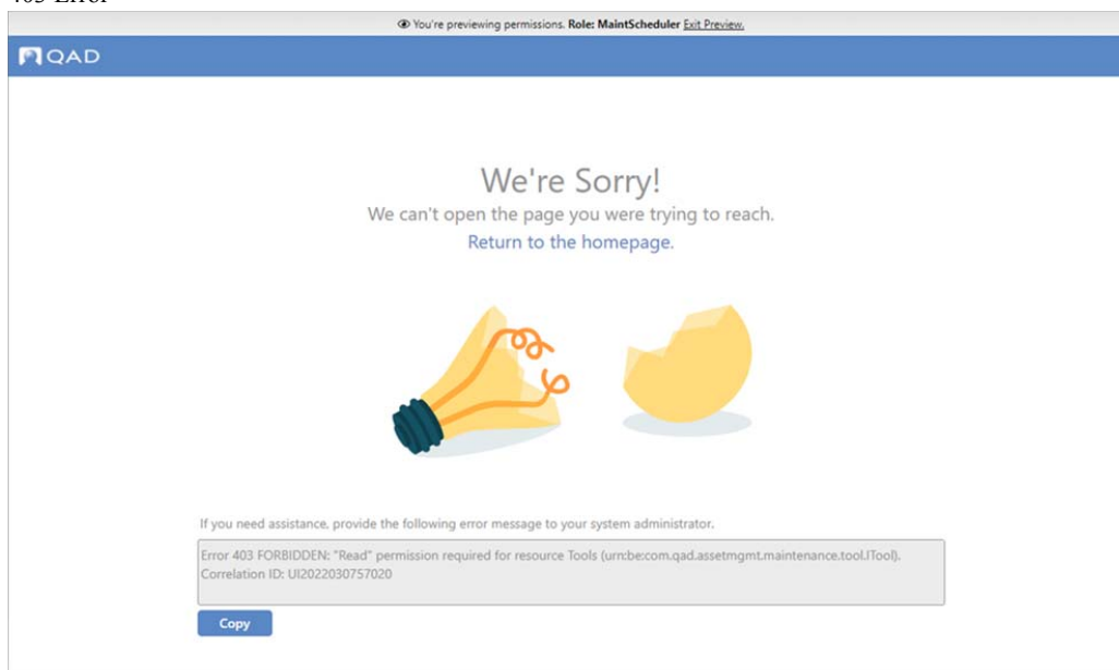
Fig. 7.19 403 Error
